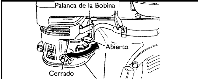
Figura 40 - Posiciones de la Bobina
