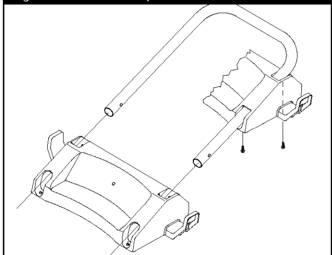
Figura 25 - Conecte Bandeja Accesorio
