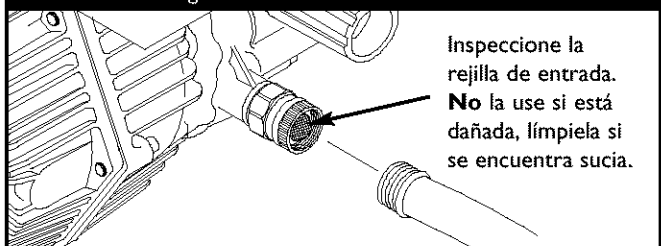
Figura 35 - Conecte la Manguera para el Jardín, a la Entrada de Agua
