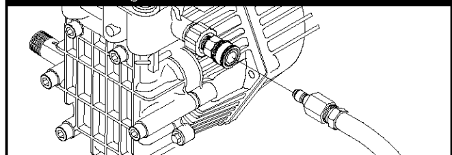
Figura 34 - Conectar la Manguera de Alta Presión a la Toma de Agua
