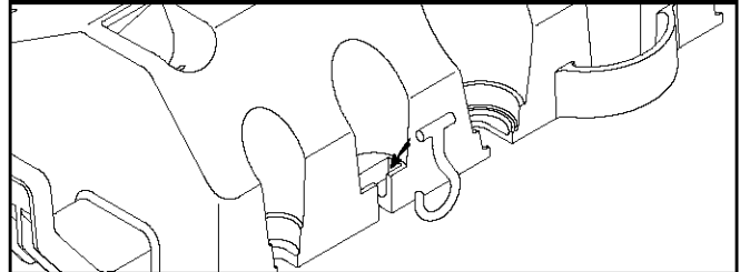
Figura 29 - Colocar el Gancho "J" Hook Sobre el Charola de Accesorios
