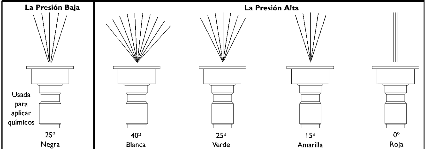
Figura 43 - Boquillas
